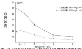
图. 单次静脉注射和单次肌肉注射氨甲环酸的药时曲线 表. 单次静脉注射和单次肌肉注射氨甲环酸的药代动力学参数
